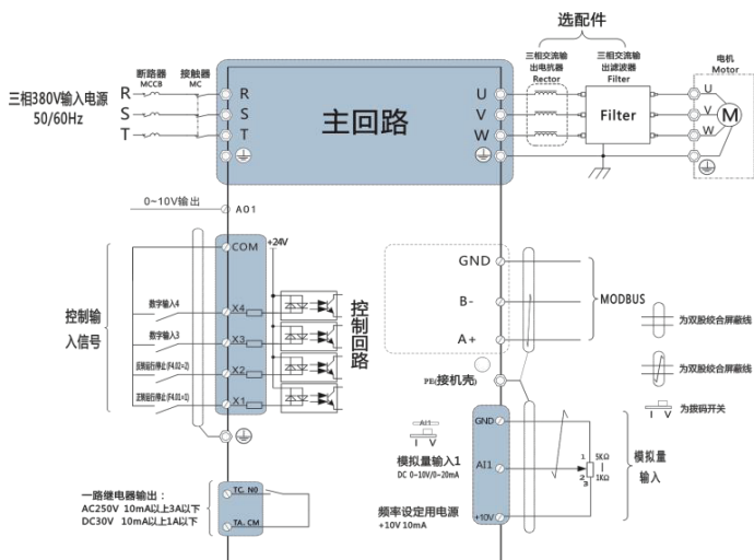
图 2-6 典型接线图
