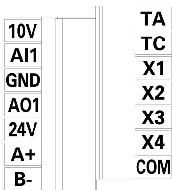
图 2-7 控制回路端子布置图
