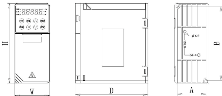
图 2-2 外形图
