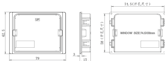
图 2-4 安装开孔尺寸图
