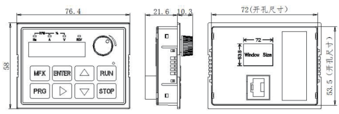
图 2-5 外形尺寸图
