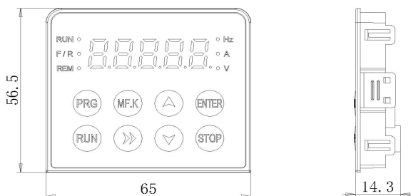
图 2-3 外形尺寸图
