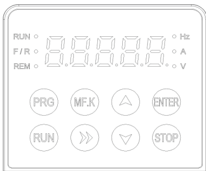
图 3-1 操作键盘布局图
